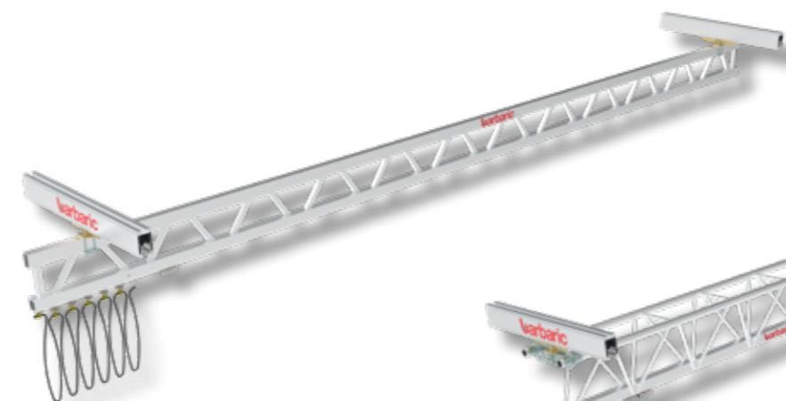
2D Alu-Fachwerksbrücke
