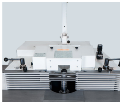
Arbre de fraiseuse Type 2620 avec joues intégrales
