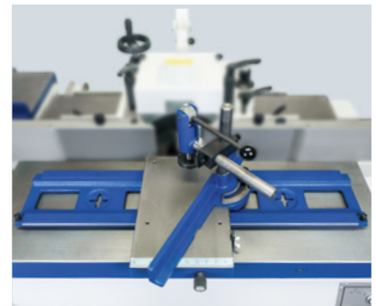
Chariot de tenonage
