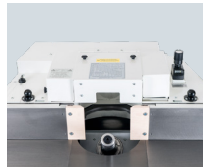
Arbre de fraiseuse Type 2620 avec AIR-LOCK et joues en acier
