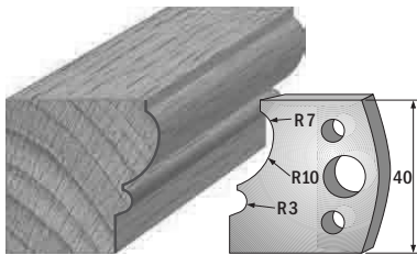
Paar Profilmesser/paire couteaux profilés 690.105 Paar Abweiser/paire limiteurs 691.105
