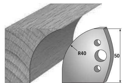
Paar Profilmesser/paire couteaux profilés 690.565 Paar Abweiser/paire limiteurs 691.565
