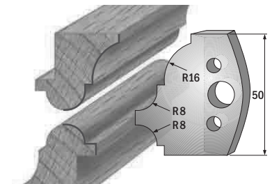
Paar Profilmesser/paire couteaux profilés 690.541 Paar Abweiser/paire limiteurs 691.541
