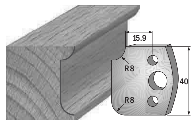
Paar Profilmesser/paire couteaux profilés 690.174 Paar Abweiser/paire limiteurs 691.174
