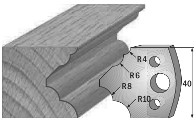
Paar Profilmesser /paire couteaux profilés 690.126 Paar Abweiser /paire limiteurs 691.126
