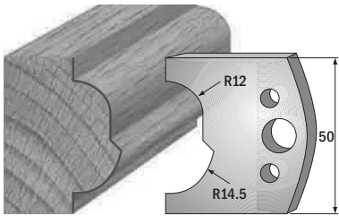
Paar Profilmesser/paire couteaux profilés 690.519 Paar Abweiser/paire limiteurs 691.519
