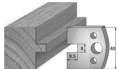
Paar Profilmesser/paire couteaux profilés 690.095 Paar Abweiser/paire limiteurs 691.095
