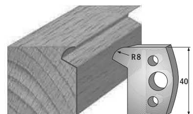
Paar Profilmesser/paire couteaux profilés 690.116 Paar Abweiser/paire limiteurs 691.116
