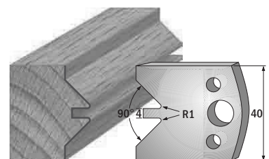
Paar Profilmesser/paire couteaux profilés 690.071 Paar Abweiser/paire limiteurs 691.071
