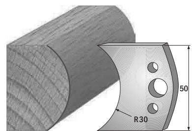
Paar Profilmesser/paire couteaux profilés 690.547 Paar Abweiser/paire limiteurs 691.547
