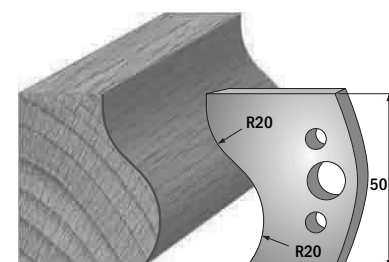
Paar Profilmesser/paire couteaux profilés 690.571 Paar Abweiser/paire limiteurs 691.571
