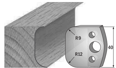
Paar Profilmesser/paire couteaux profilés 690.050 Paar Abweiser/paire limiteurs 691.050
