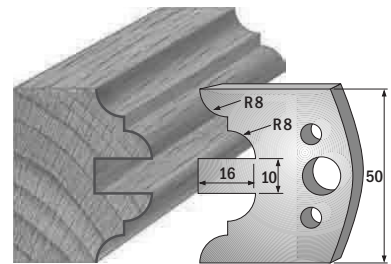
Paar Profilmesser/paire couteaux profilés 690.522 Paar Abweiser/paire limiteurs 691.522
