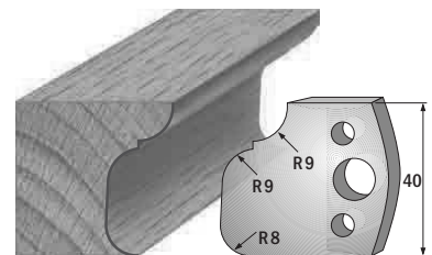
Paar Profilmesser/paire couteaux profilés 690.068 Paar Abweiser/paire limiteurs 691.068
