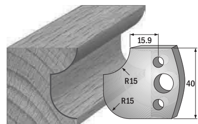
Paar Profilmesser/paire couteaux profilés 690.177 Paar Abweiser/paire limiteurs 691.177
