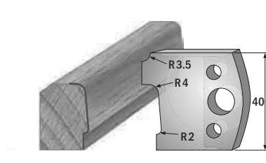
Paar Profilmesser /paire couteaux profilés 690.130 Paar Abweiser /paire limiteurs 691.130
