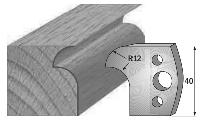
Paar Profilmesser/paire couteaux profilés 690.005 Paar Abweiser/paire limiteurs 691.005
