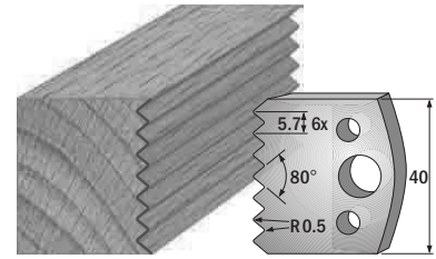
Paar Profilmesser/paire couteaux profilés 690.077 Paar Abweiser/paire limiteurs 691.077
