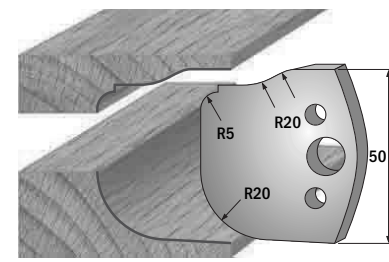
Paar Profilmesser/paire couteaux profilés 690.577 Paar Abweiser/paire limiteurs 691.577
