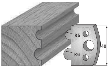
Paar Profilmesser/paire couteaux profilés 690.030 Paar Abweiser/paire limiteurs 691.030
