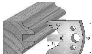
Paar Profilmesser/paire couteaux profilés 690.098 Paar Abweiser/paire limiteurs 691.098
