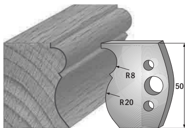
Paar Profilmesser/paire couteaux profilés 690.502 Paar Abweiser/paire limiteurs 691.502
