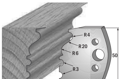
Paar Profilmesser/paire couteaux profilés 690.513 Paar Abweiser/paire limiteurs 691.513
