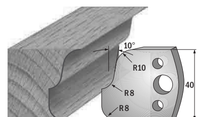
Paar Profilmesser/paire couteaux profilés 690.059 Paar Abweiser/paire limiteurs 691.059
