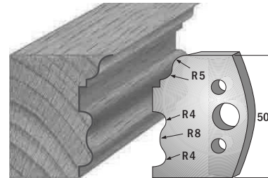
Paar Profilmesser/paire couteaux profilés 690.515 Paar Abweiser/paire limiteurs 691.515
