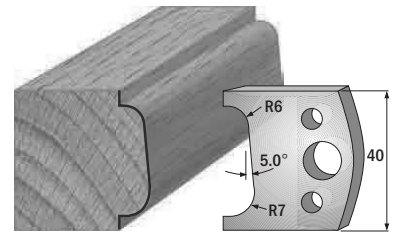
Paar Profilmesser/paire couteaux profilés 690.002 Paar Abweiser/paire limiteurs 691.002
