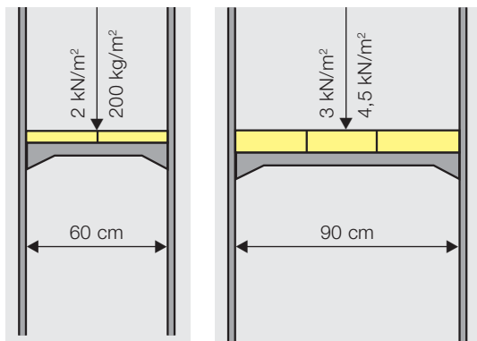
Bild 3: Verputz-/Malergerüst.
