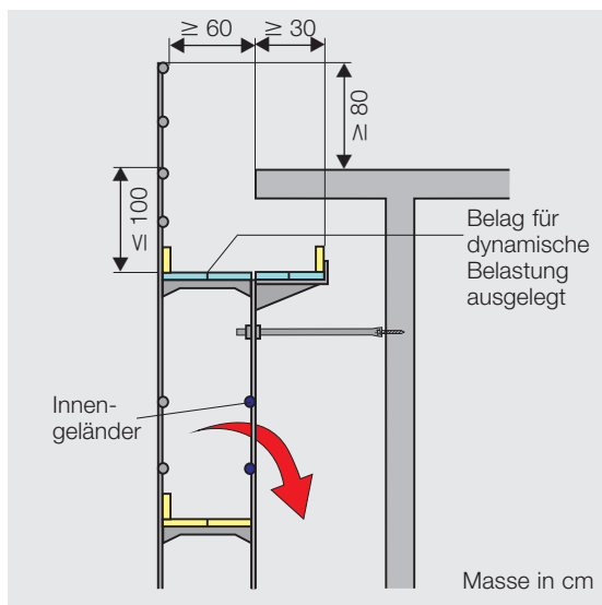
Bild 20: Spenglergang.
