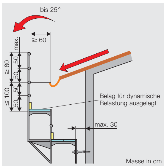
Bild 22: Seitenschutz eines Spenglergangs bei einer Dachneigung bis 25°.
