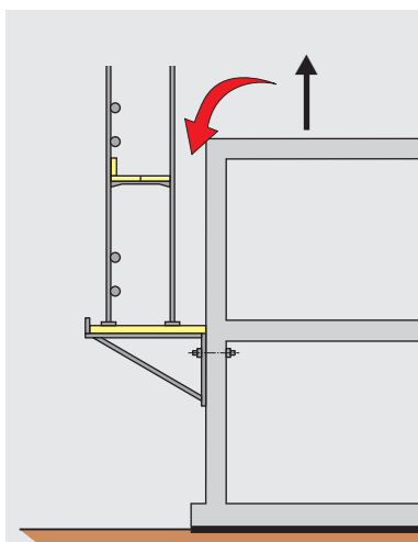
Bild 8: Konsolgerüst.
