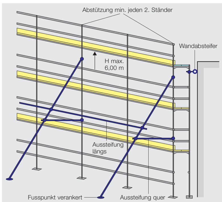
Bild 18: Aussenabstützung anstelle von Verankerungen.
