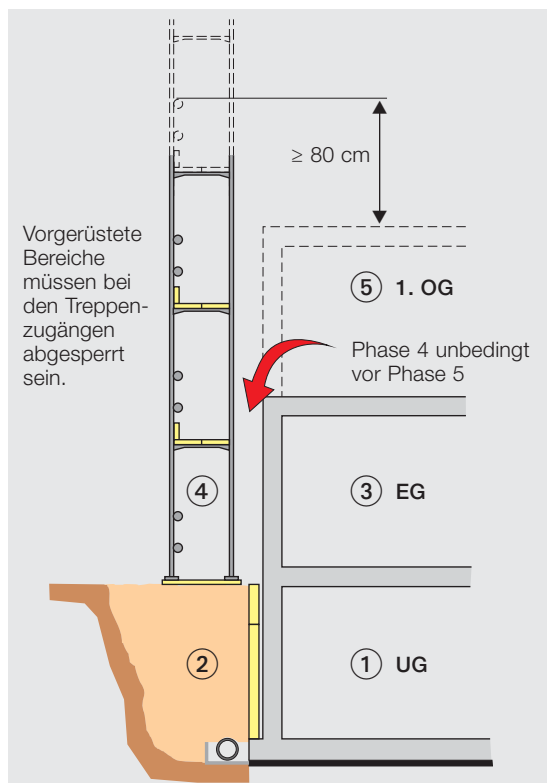
Bild 6: Vorgehensschritte ① bis ⑤.
