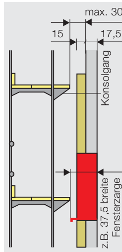
Bild 14: Konsolgänge.
