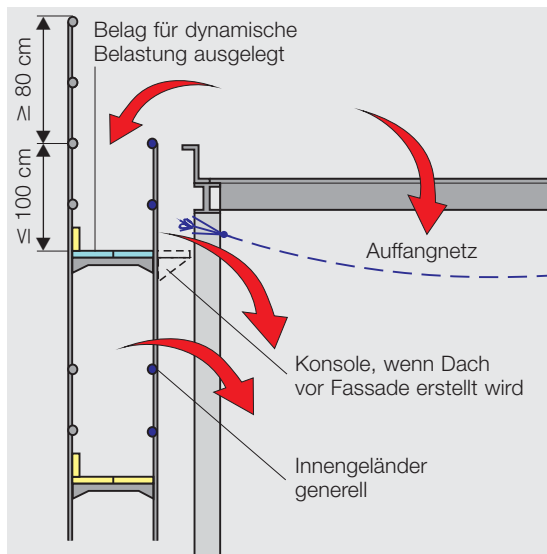
Bild 25: Montagebau.
