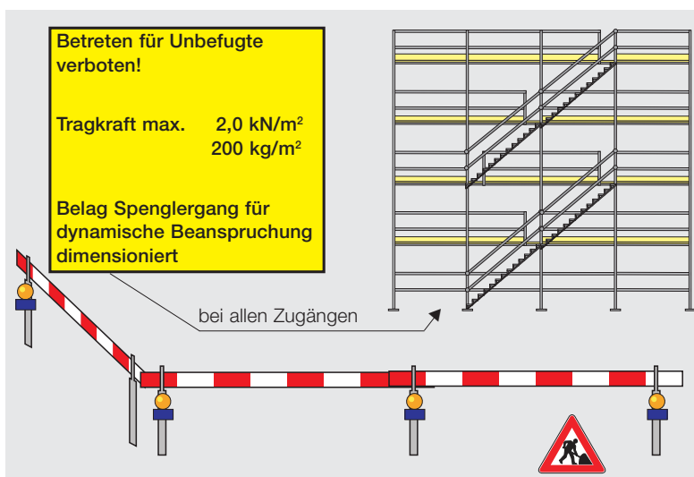
Bild 5: Die Nutzlast eines Arbeitsgerüsts muss (bei den Zugängen) auf einem Schild gut sichtbar angegeben sein.
