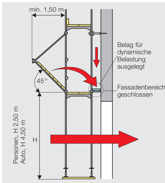
Bild 28: Schutz bei Durchgängen.
