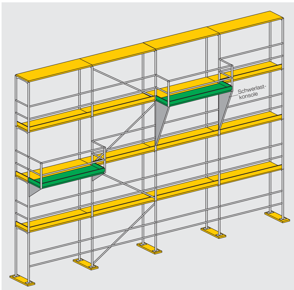
Bild 27: Versetzte Podeste für den Materialumschlag.
