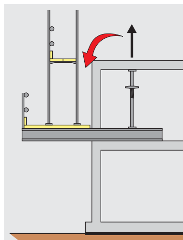
Bild 9: Auslegergerüst.
