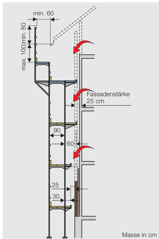
Bild 11: Nachträglich hochgezogenes Putzmauerwerk.
