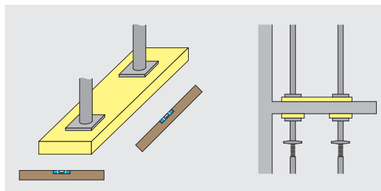
Bild 7: Konventionelle Fundamente.
