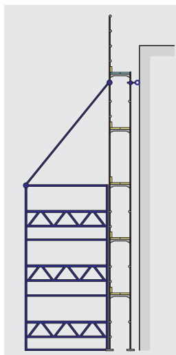
Bild 19: Beispiel Aussenabstützung mit querstehenden Gerüstfeldern.
