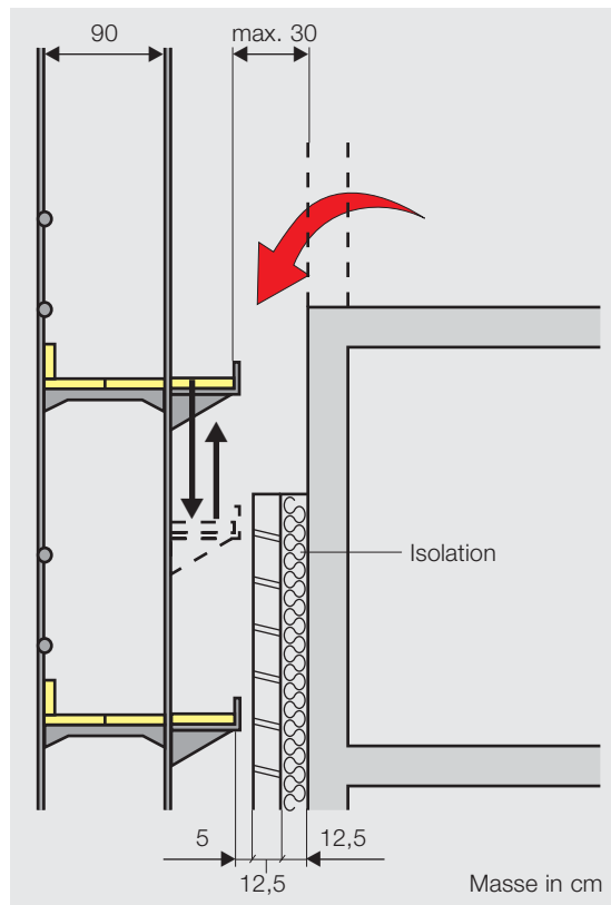
Bild 10: Nachträglich hochgezogenes Sichtmauerwerk.
