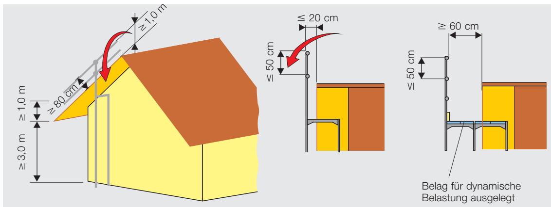
Bild 24: Giebelseitiger Seitenschutz.
